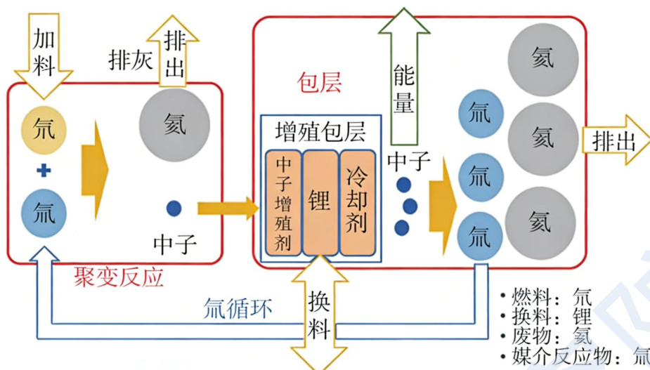
图 2 聚变主循环原理示意图
